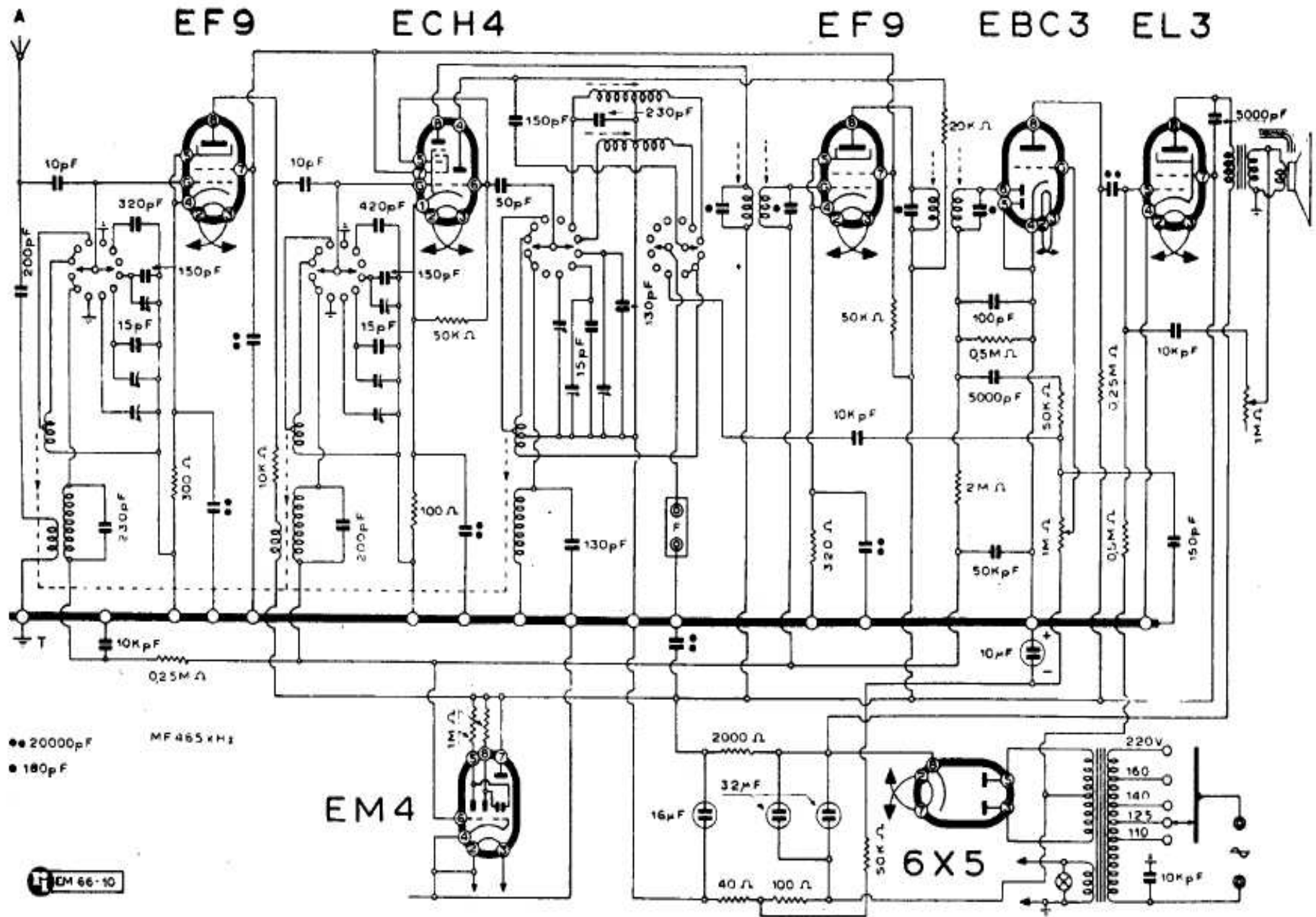
A.B.C. RADIOCOSTRUZIONI - Mod. R 962
